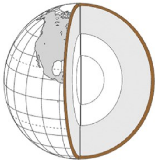
Земна кора
