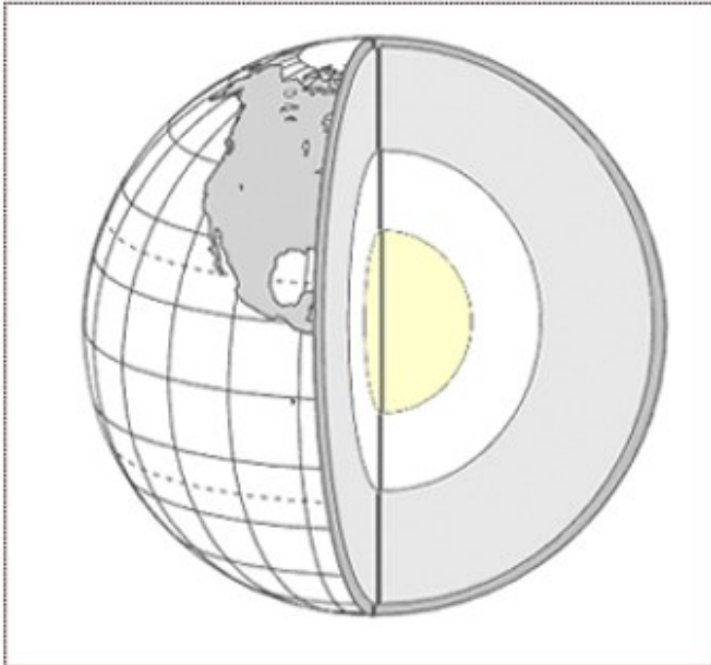
Вътрешно ядро
