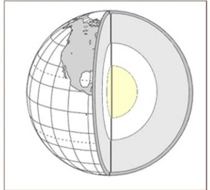
Вътрешно ядро
