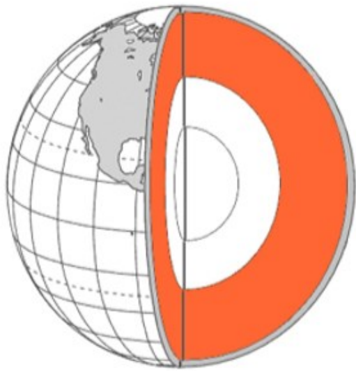
Земна мантия
