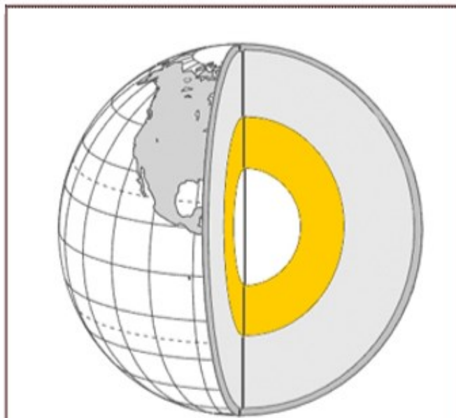
Външно ядро
