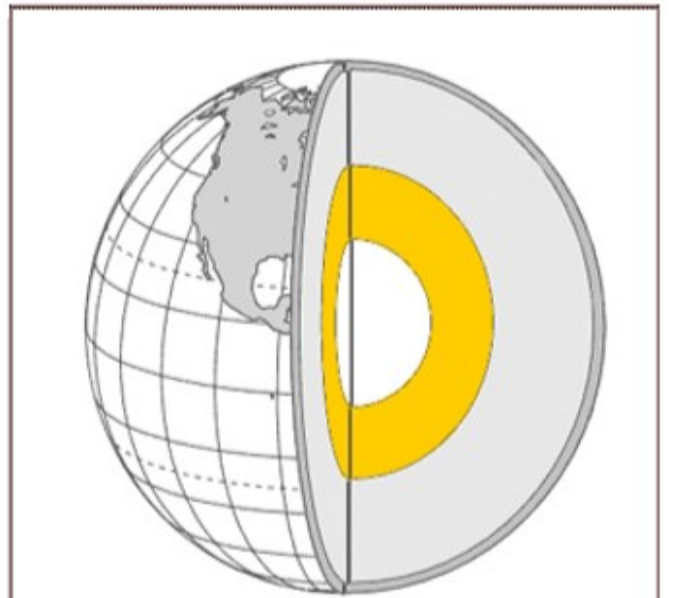
Външно ядро
