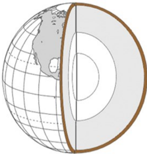
Земна кора
