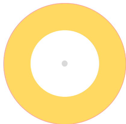
Външно ядро
