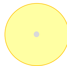
Вътрешно ядро
