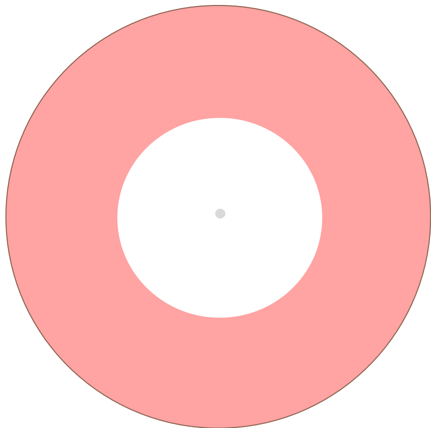
Земна мантия
